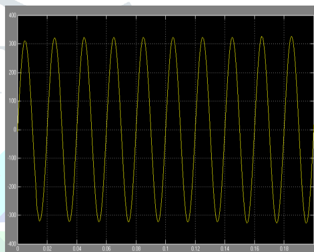
Fig. 6. Load voltage
