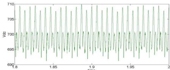
Fig. 6 DC link voltage.
