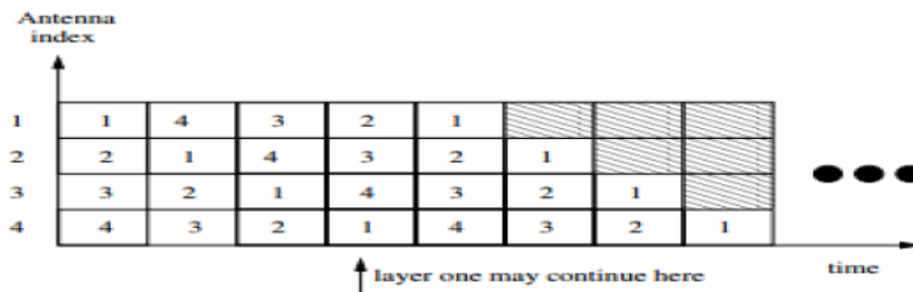
Fig 1.4.4.1: D-BLAST layer diagram
