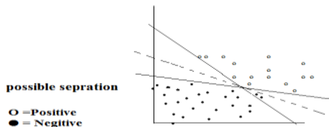
Fig 3: Linear Classifier
