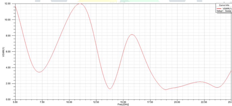
Fig. 9 VSWR
