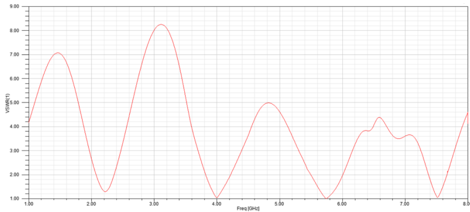
Fig. 9 VSWR
