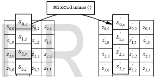
Fig: D-Mix column transformation
