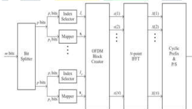
Fig. 2: OFDM IM Transmitter Block Diagram
