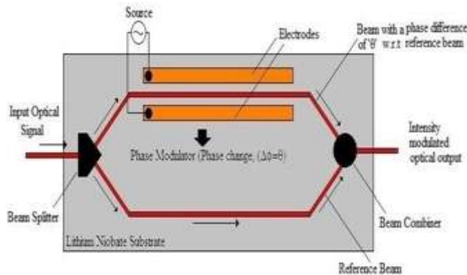
Fig. 2. Mach-Zehnder Interferometer
